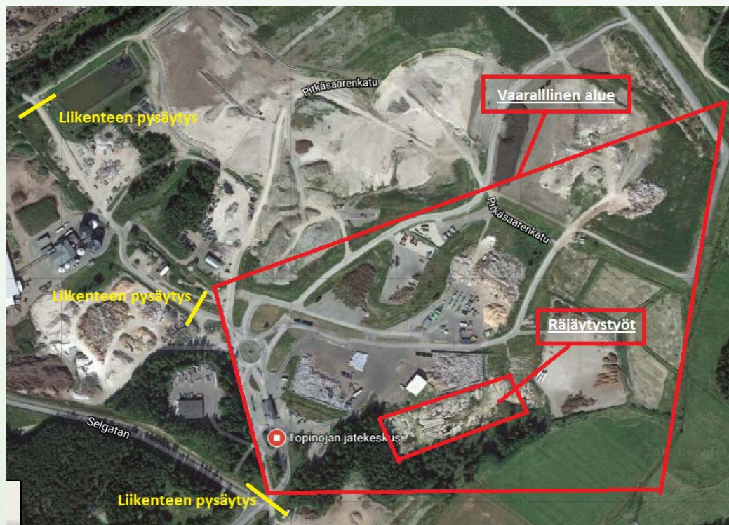
Räjäytystöiden aikainen vaara-alue ja liikenteen pysäytyspaikat.
